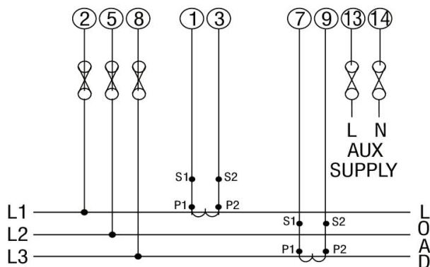
b) 3 Phase 3 Wire
