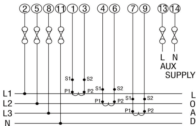
a) 3 Phase 4 Wire
